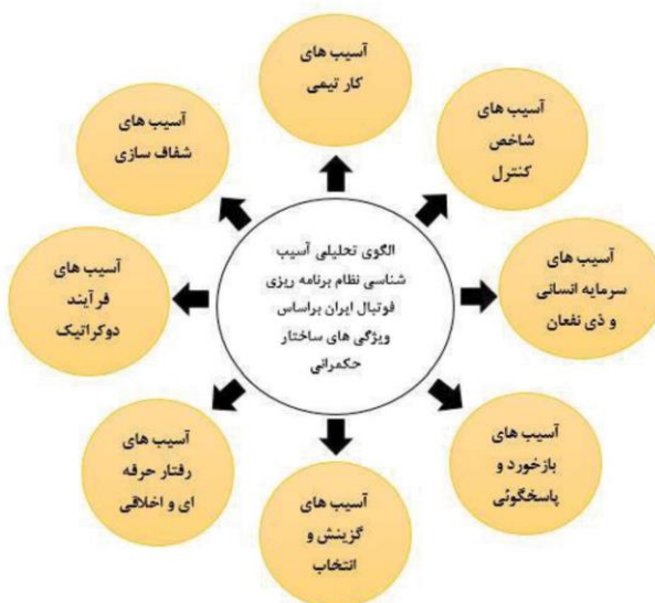
شکل ۱. الگوی تحلیلی آسیب شناسی نظام برنامه ریزی فوتبال ایرن بر اساس ویژگی های ساختار حکمرانی
