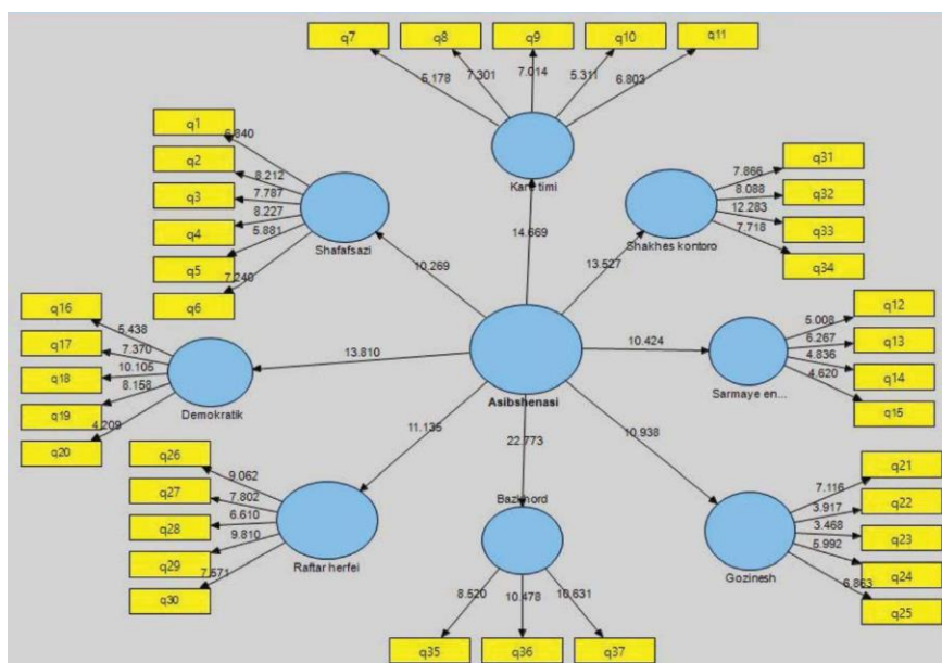
شکل ۳. مدل تحقیق در حالت شاخص
